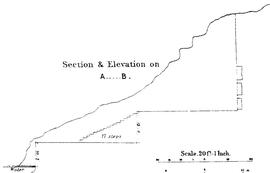
تصویر شماره ۵: مقطع اثر صخره‌ای قدمگاه، ترسیم: H.L.wells, Proc.R.G.S,V,1883, fig.p:184 (اقتباس از: Boucharlat, Iranica Antiqua, 1979, P:156)
