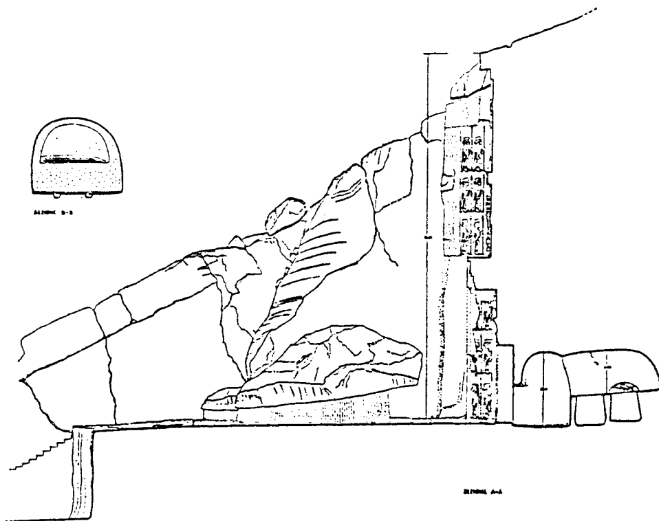
تصویر شماره ۱۰: نقشه (پلان) و مقطع آرامگاه صخره‌ای اردشیر سوم (واقع در تخت جمشید) (اقتباس از: Boucharlat, Iranica Antiqua, 1979, P:162)
